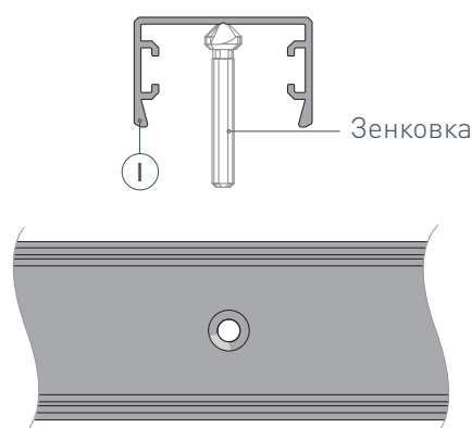
Рис. 1. Профиль ① со снятой фаской, вид снизу
