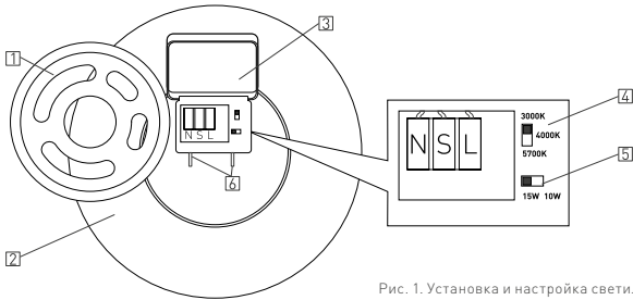
Рис. 1. Установка и настройка светильника
