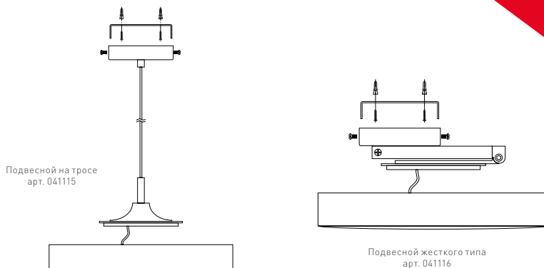
Рис. 2. Установка светильника с использованием дополнительных аксессуаров
