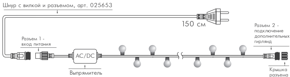
Рисунок 1. Схема подключения.
