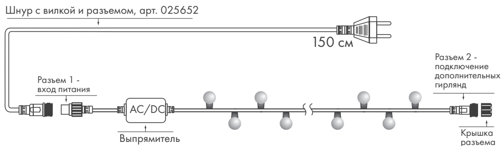
Рисунок 1. Схемы подключения.
