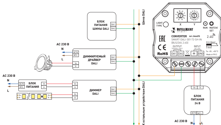
Рис. 1. Схема подключения конвертера
