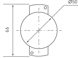
Рисунок 2. Чертеж модуля
