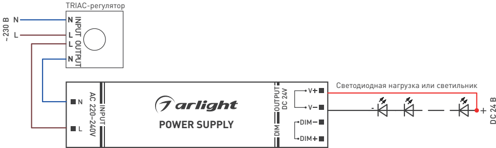
Рис. 1. Пример подключения источника питания с TRIAC-регулятором
