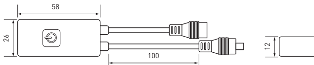
Рис. 1. Габаритный чертеж
