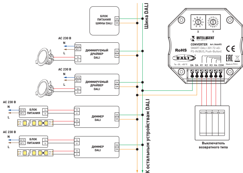
Рис. 1. Схема подключения конвертера
